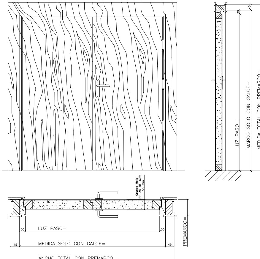
PUERTA DE MADERA CORTAFUEGOS 2 H
